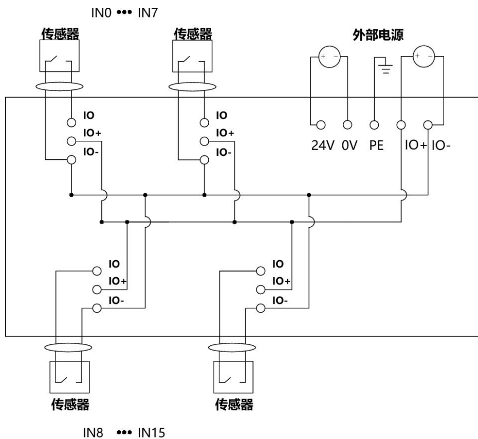
(2) RX2EC-1600-N-4/5 接线图
