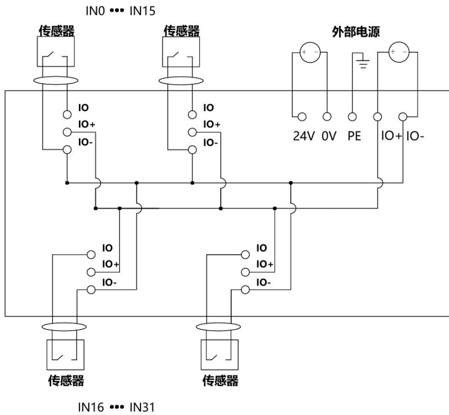
(4) RX2EC-3200-N-4/5 接线图
